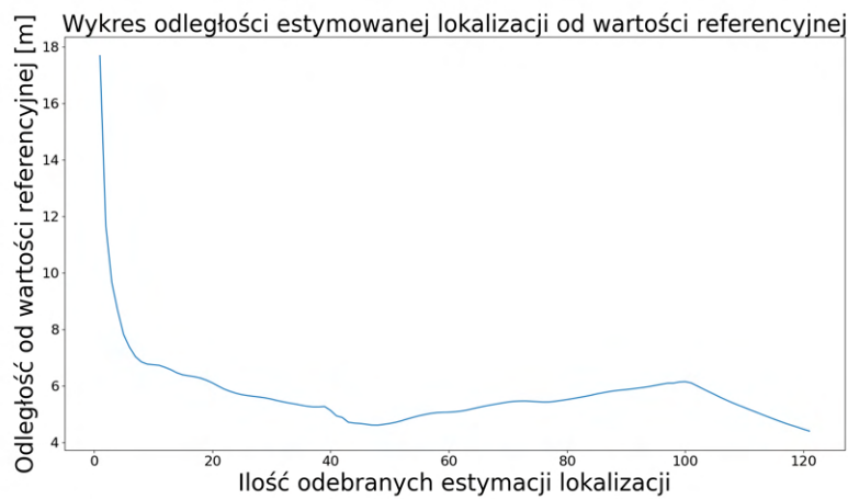
Rysunek 4.11: Wykres prezentujący odległość estymacji lokalizacji obiektu w środowisku produkcyjnym od punktu referencyjnego.
