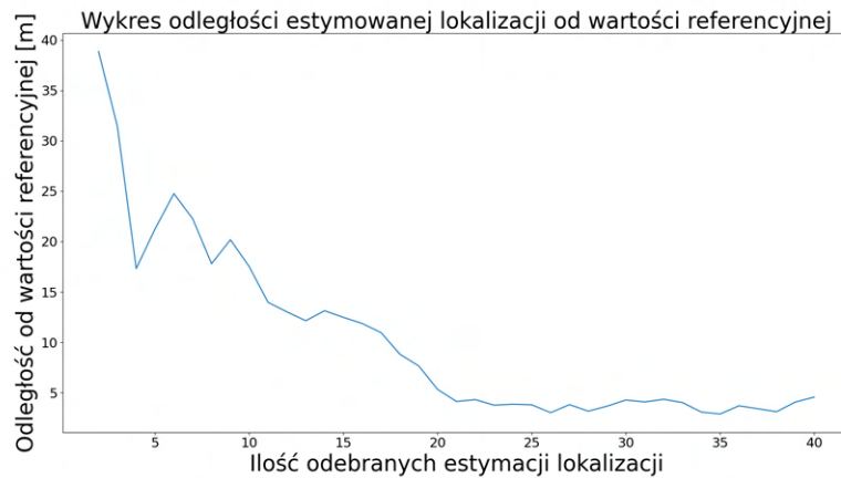
Rysunek 4.7: Wizualizacja estymacji odległości lokalizacji od wartości referencyjnej dla danych testowych podczas jednej z przeprowadzonych symulacji.
