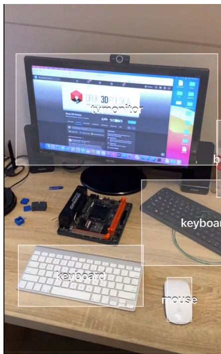
Rysunek 4.2: Przykład detekcji obiektów z poziomu aplikacji uruchomionej na smartfonie z systemem iOS (uruchomionej w trybie Debug- użytkownik końcowy nie widzi (bounding boxów))
